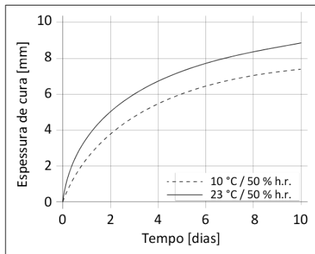
Diagrama 1: Velocidade de cura do Sikaflex®-292i
