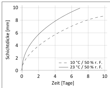
Diagramm 1: Durchhärtengeschwindigkeit Sikaflex®-296
