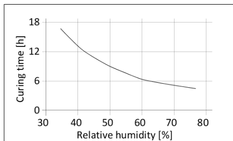
Diagramm 1: Durchhärtungszeit für einen 500 µm Klebstofffilm
