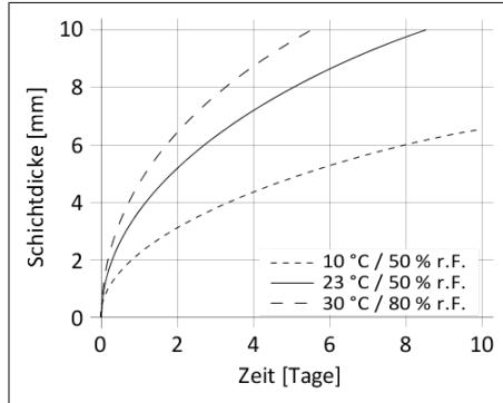
Diagramm 1: Durchhärtgeschwindigkeit von Sikaflex®-254
