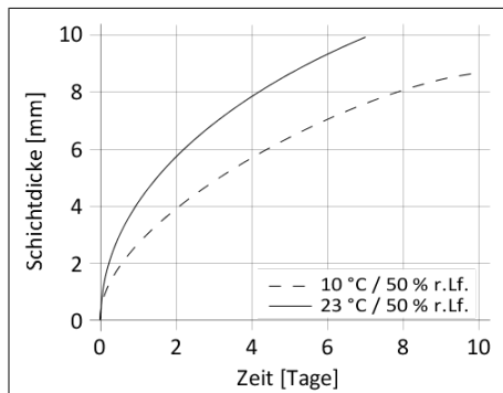
Diagramm 1: Durchhärtegeschwindigkeit SikaTack®-MOVE Transportation
