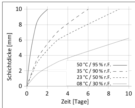
Diagramm 1: Durchhärtgeschwindigkeit Sikasil® AS-70
