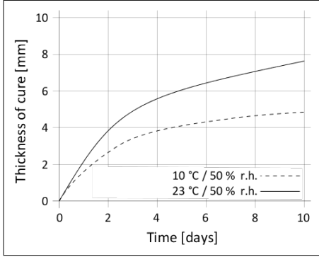
Dijagram 1: Brzina stvrdnjavanja Sikaflex®-521 UV
