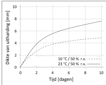
Schema 1: Uithardingsnelheid Sikaflex®-521 UV
