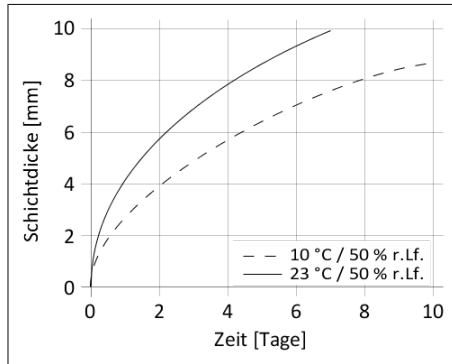
Diagramm 1: Durchhärtengeschwindigkeit
