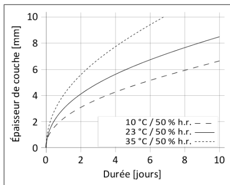
Diagramme 1: Vitesse de durcissement de Sikaflex®-554
