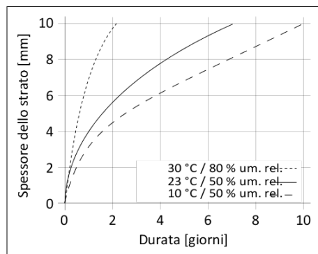
Diagramma 1: velocità di polimerizzazione di Sikaflex®-645
