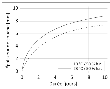
Diagramme 1: Vitesse de durcissement de Sikaflex®-292i
