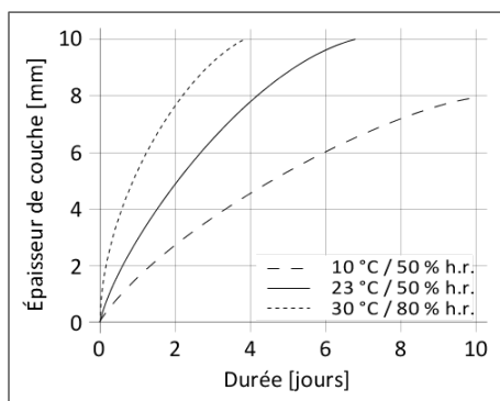
Diagramme 1: Vitesse de durcissement SikaTack® Panel-50
