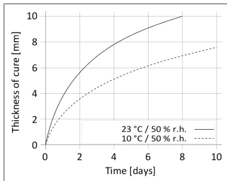
Diagram 1: Rychlost vytvrzení Sikaflex®-291i
