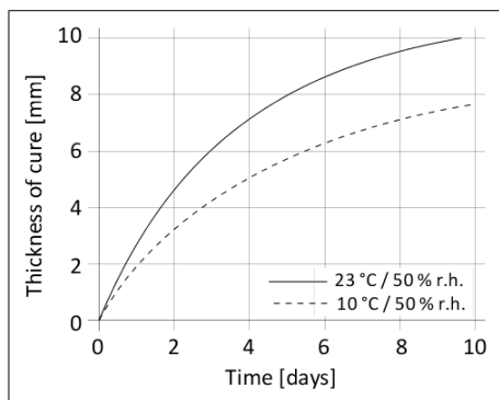
Graf 1: Rychlost vytvrzování Sikaflex®-515
