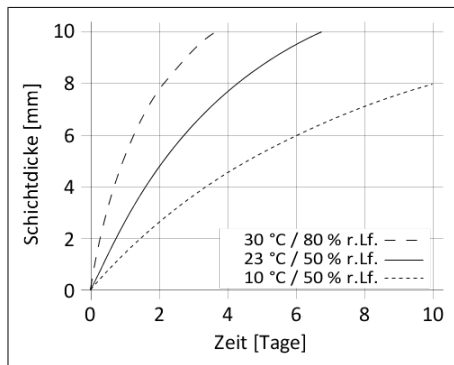
Diagramm 1: Durchhärtengeschwindigkeit Sikaflex®-268
