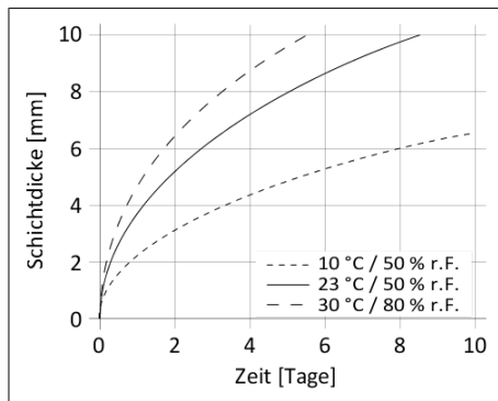
Diagramm 1: Durchhärtgeschwindigkeit von Sikaflex®-254
