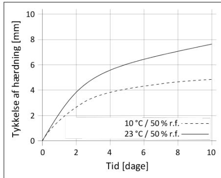
Diagram 1: Hærdningshastighed Sikaflex®-521 UV
