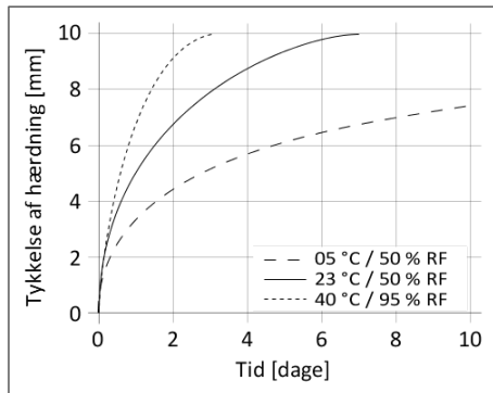
Diagram 1: Hærdehastighed Sikasil® WS-605 S
