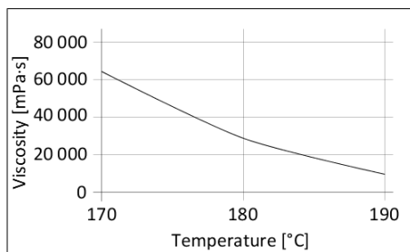
Diagrama 1: Viscosidad como función de la temperatura
