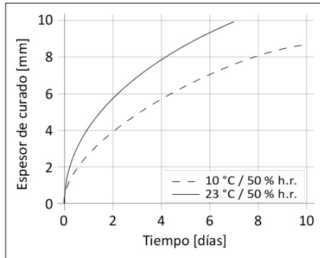
Diagrama 1: Velocidad de curado para SikaTack® PRO
