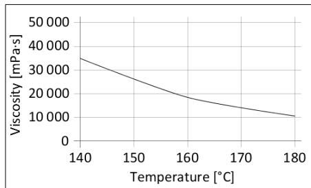
Diagrama 1: Viscosidad en función de la temperatura.
