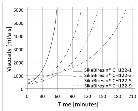
Diagramme 2: Développement de la viscosité à 25 °C
