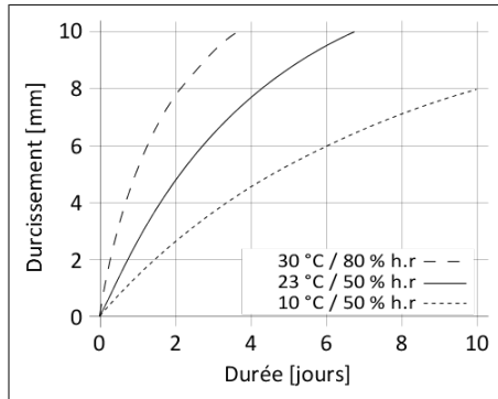
Diagramme 1 : Vitesse de polymérisation du Sikaflex®-252
