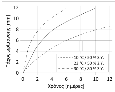
Διάγραμμα 1: Ταχύτητα ωρίμανσης Sikaflex®-252
