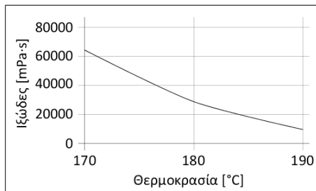
Διάγραμμα 1: Το ιξώδες σε συνάρτηση με τη θερμοκρασία. Κατά τη διακοπή εργασιών, το SikaMelt®-285 πρέπει να επεξεργαστεί ως ακολούθως:
