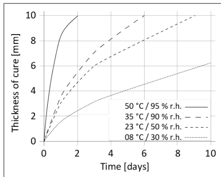
Διάγραμμα 1: Ταχύτητα ωρίμανσης Sikasil® AS-70
