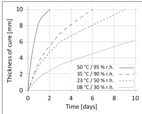
Διάγραμμα 1: Ταχύτητα ωρίμανσης σιλικονών Sikasil® SG-20
