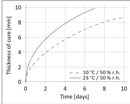
Διάγραμμα 1: Ταχύτητα ωρίμανσης του Sikaflex®-227
