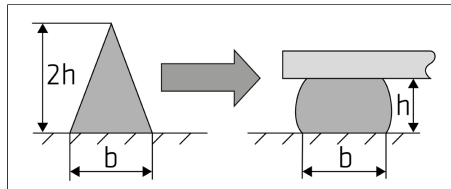
Εικόνα 1: Συνιστώμενος τρόπος διαμόρφωσης τριγωνικού κορδονιού
