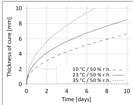
Diagramma 1: Velocità di indurimento di Sikaflex®-554
