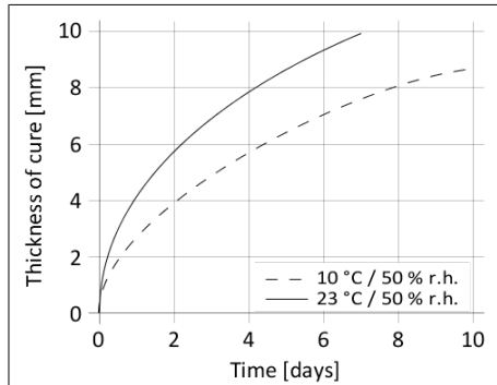
Diagramma 1: Velocità di indurimento per SikaTack® MOVE Transportation
