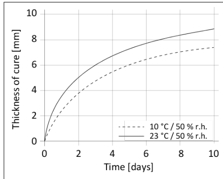
Diagrama 1: Velocidad de curado de Sikaflex®-292i
