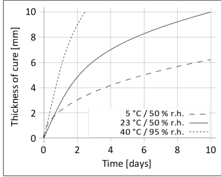
Diagrama 1: Velocidad de curado de Sikasil® SG-20 S
