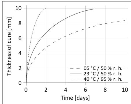
Diagrama 1: Velocidade de cura do Sikasil® WS-300 EU
