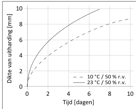
Figuur 1: doorhardingsnelheid van Sikaflex®-265
