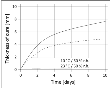
Diagram 1: Uithardingsssnelheid Sikaflex®-529 Evolution
