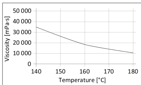
Wykres 1: Lepkość w zależności od temperatury
