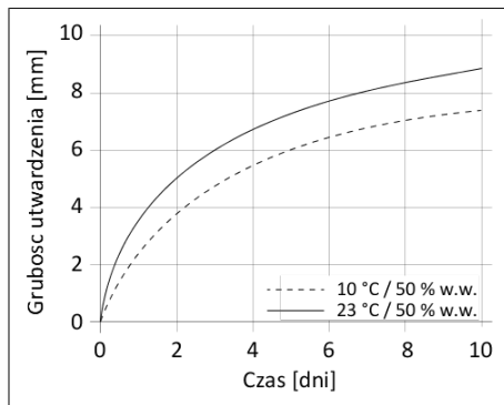
Wykres 1: Szybkość utwardzania Sikaflex®-292i
