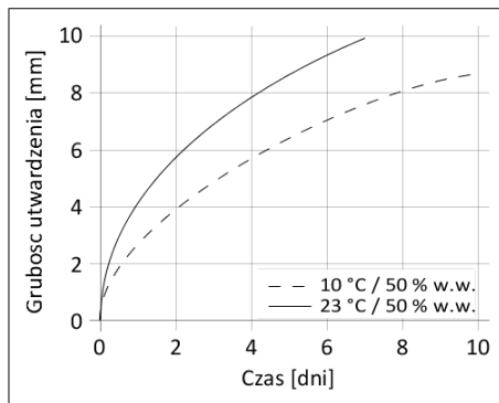
Wykres 1: Szybkość utwardzania Sikaflex®-265
