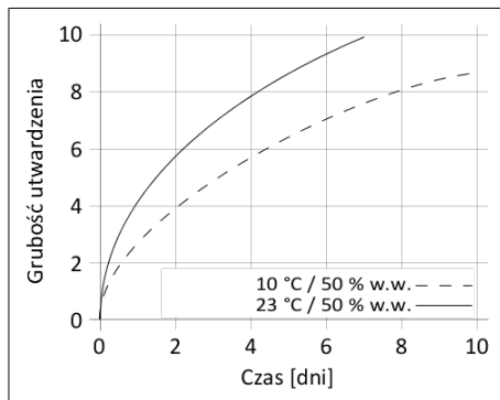
Wykres 1: Szybkość utwardzania SikaTack® PRO (Purform®)
