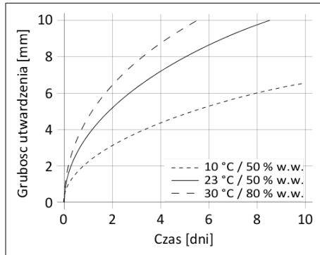
Wykres 1: Szybkość utwardzania Sikaflex®-254
