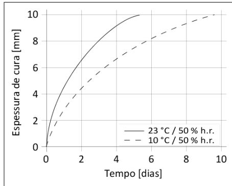
Diagrama 1: Velocidade de cura Sikaflex®-298
