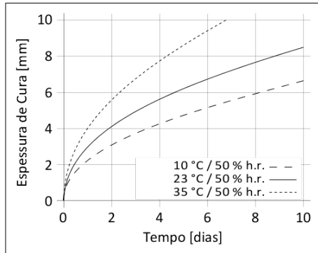
Diagrama 1: Velocidade de cura de Sikaflex®-554
