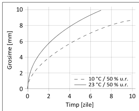
Diagrama 1: Viteza de întărire pentru Sikaflex®-223
