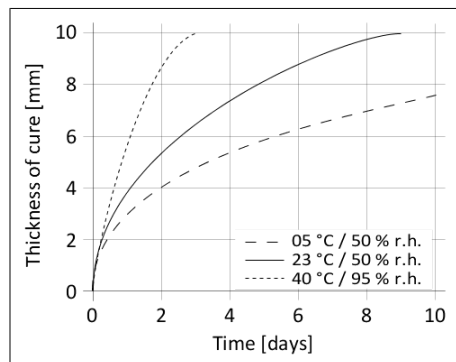
Graf 1: Rýchlosť vytvrdzovania Sikasil® WS-200
