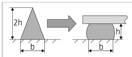
Obrázok 1: Odporúčany dizajn nánosu lepidla
