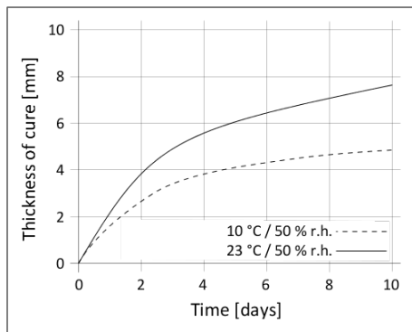
Діаграма 1: Швидкість полімеризації Sikaflex®-522
