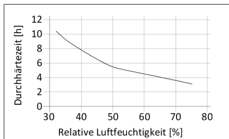
Diagramm 1: Durchhärtezeit für einen 500 µm Klebstofffilm
