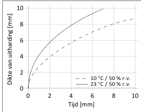
Schema 1: Uithardingsnelheid SikaTack® PRO
